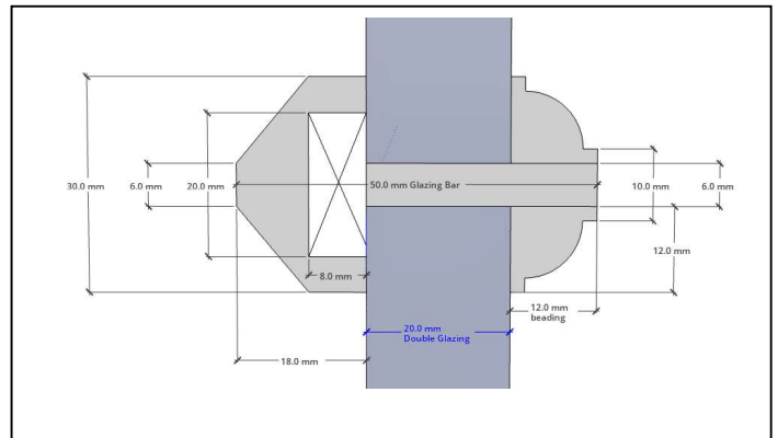
Glazing Bar
